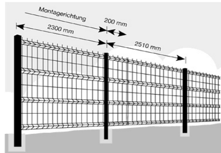
Pfostenabstand
